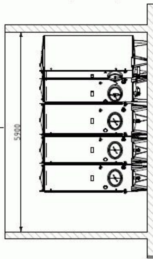
C-C ( 1 : 50 )
