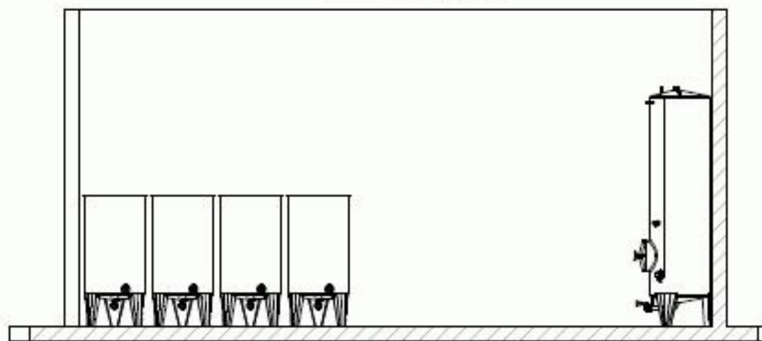
B-B ( 1 : 50 )
