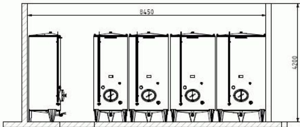
A-A ( 1 : 50 )
