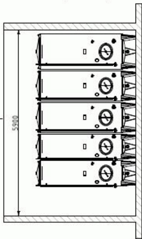
C-C ( 1 : 50 )
